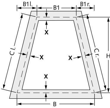
Bestellmaße = B, B1, B1 l., B1 r. und H
