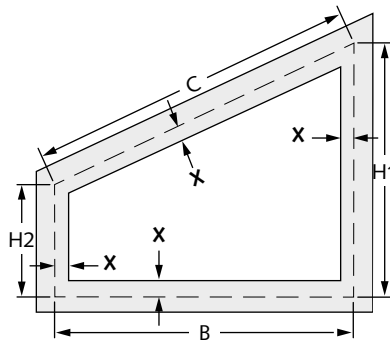
Bestellmaße = B, H1 und H2
