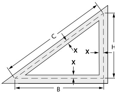
Bestellmaße = B und H
