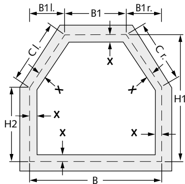
Bestellmaße = B, B1, B1 l., B1 r., H1 und H2
