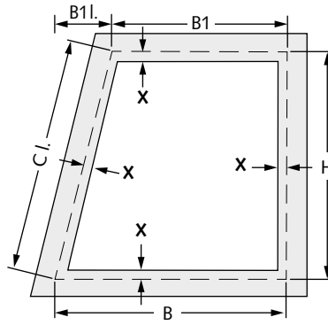
Bestellmaße = B, B1, B1 l.(r.) und H
