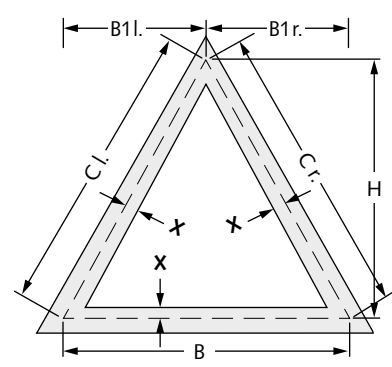
Bestellmaße = B, B1 l., B1 r. und H
