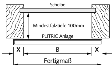
Bestellmaße = B, B1, B1 l., B1 r., H1 und H2
