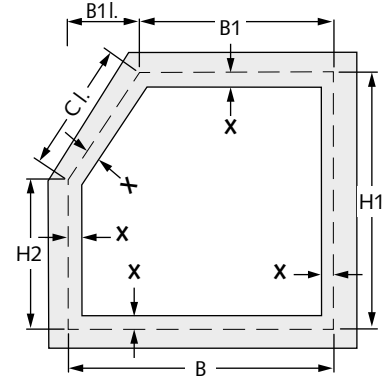
Bestellmaße = B, B1, B1 l.(r.), H1 und H2
